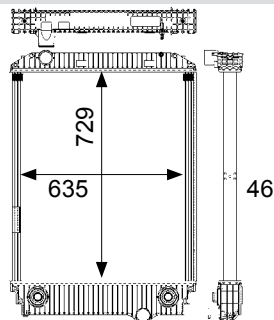
376753311 Radiator
